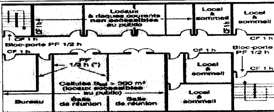
Niveau cloisonné traditionnellement (bâtiment SF 1 h).
